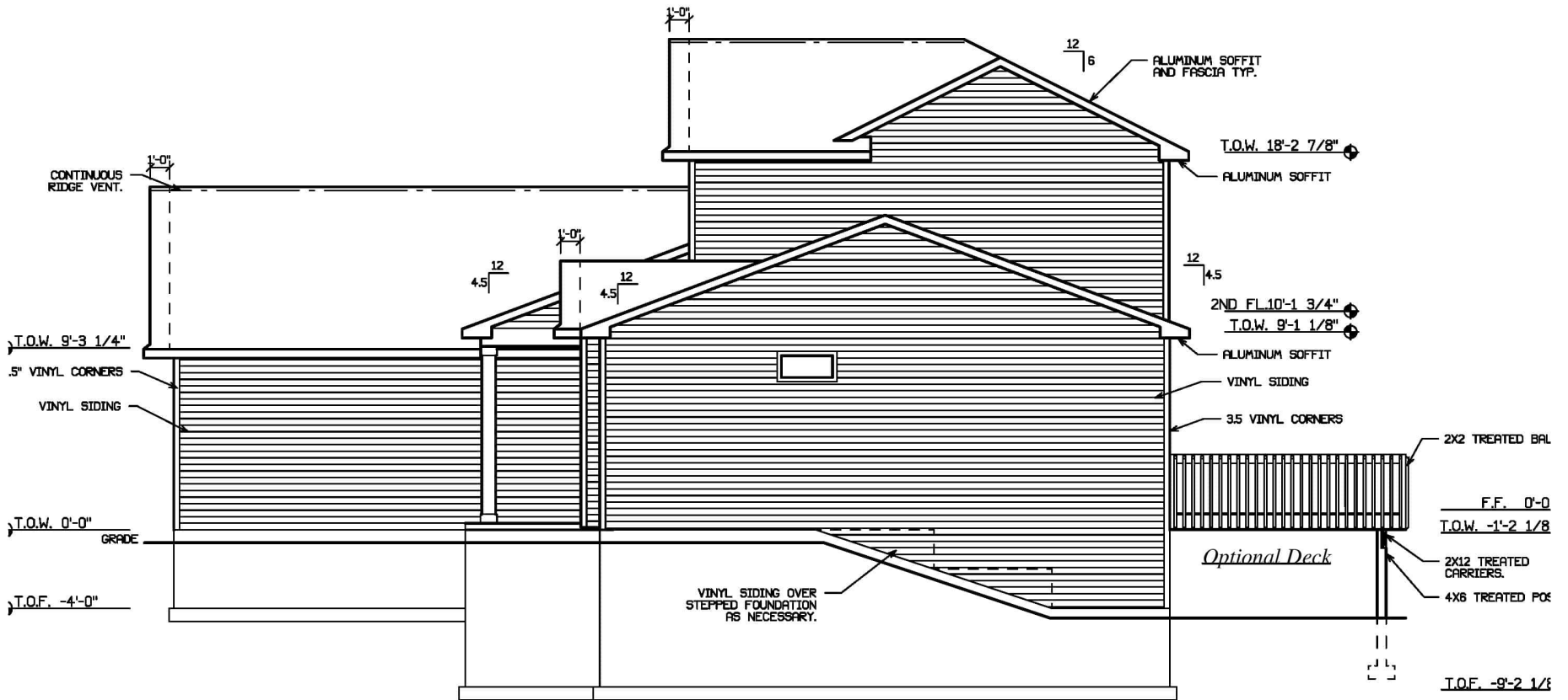
Right Elevation
