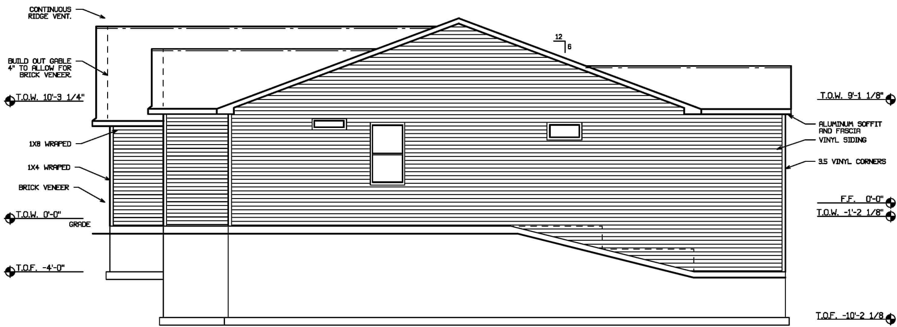
Right Elevation
